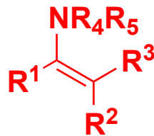
Enamine
