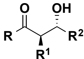
Anti -aldol
