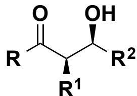
Syn -aldol
